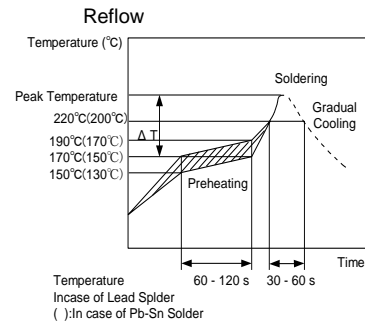
Vapor Reflow
